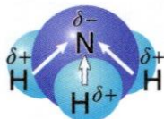
アンモニア \text{NH}_3
