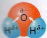
水 \text{H}_2\text{O}
