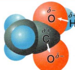
酢酸 3 \text{CH}_3\text{COOH}
