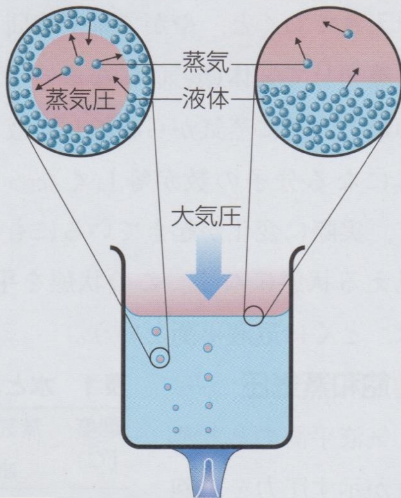
図 12 液体の沸騰
