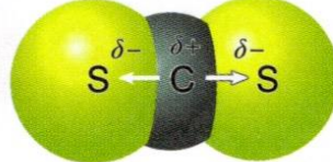
二硫化炭素 \text{CS}_2
