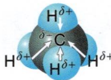
メタン \text{CH}_4
