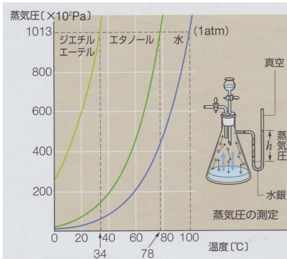
図 10 蒸気圧曲線
