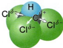
クロロホルム 3 \text{CHCl}_3
