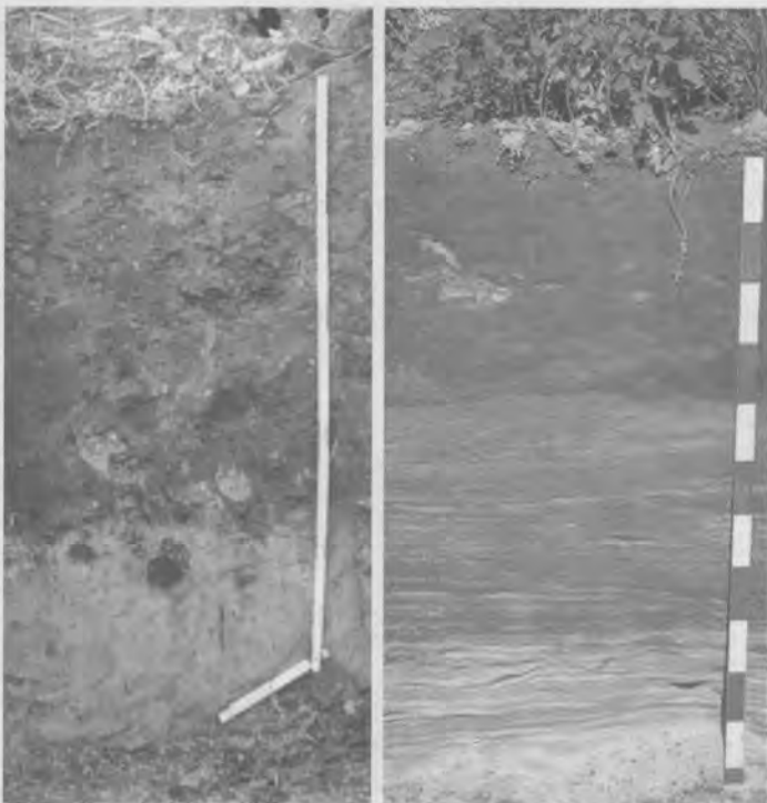
典型的なチェルノーゼム土壌断面(左)と黒ボク土壌断面(右)
